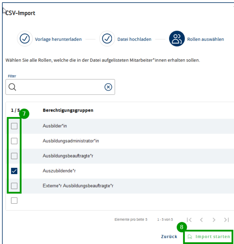
Abbildung 19: CSV-Import starten
